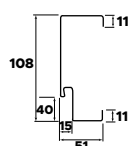
Rysunek techniczny
