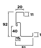
Rysunek techniczny
