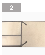
Skrzydło drzwiowe z uszczelką, wypełnione pianką poliuretanową oraz ramiakiem z kompozytu z włókna szklanego z strukturą karbonu
